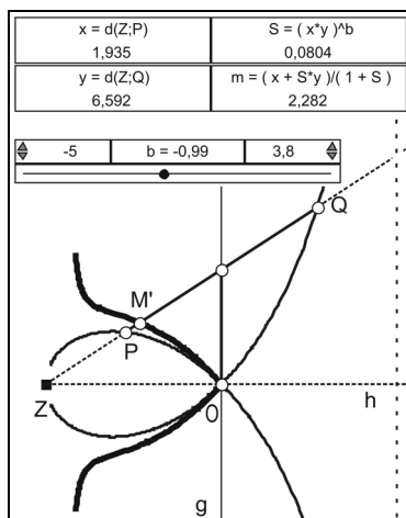
Abb. 29: strophoidale Darstellung für ein weiteres erfundenes Mittel
