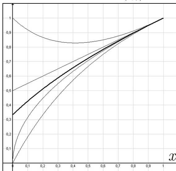
Abb. 9: Darstellung einer willk\u00fcrlich erzeugten Mittelwertfunktion als Einbettung in Abb. 4 (rechts)
