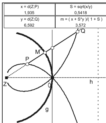
Abb. 25: strophoidale Darstellung für das geometrische Mittel
