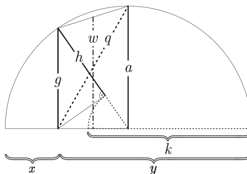
Abb. 15: Mittelwertdarstellung in Erweiterung der Darstellung nach Pappus
