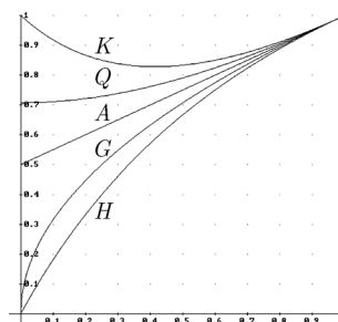
Abb. 13: quadratisches Mittel zwischen vier pythagoreischen Mittelwerten
