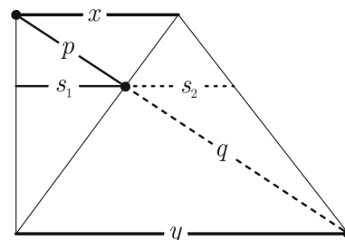
Abb. 17: Zum Beweis, dass die Mittellinie durch den Diagonalenschnittpunkt das harmonische Mittel darstellt.
