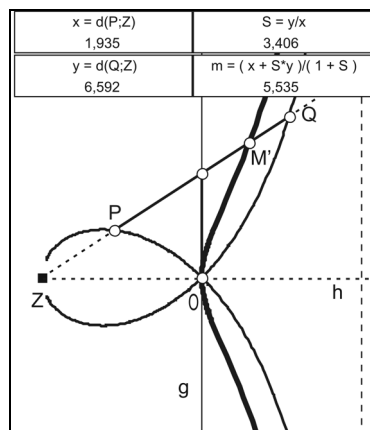
Abb. 26: strophoidale Darstellung für das kontraharmonische Mittel
