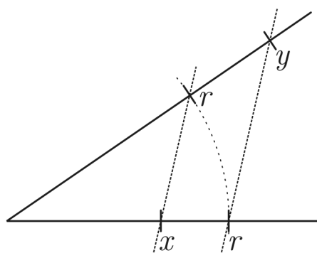
Abb. 11: geometrisches Mittel mittels Strahlensatz – wie erhält man r ?
