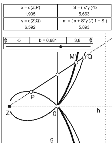
Abb. 28: strophoidale Darstellung für ein erfundenes Mittel
