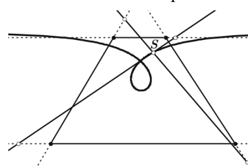
Abb. 22: Variation von Abb. 21: Ausgangsfigur ist ein symmetrisches Trapez
