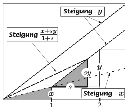
Abb. 8: Chuquetmittel von x und y ?
