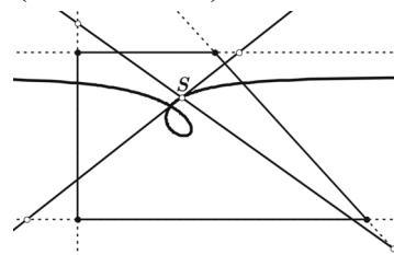
Abb. 21: Ortslinie des variierten Schnittpunkts bei Zulassung auch äußerer Teilpunkte
