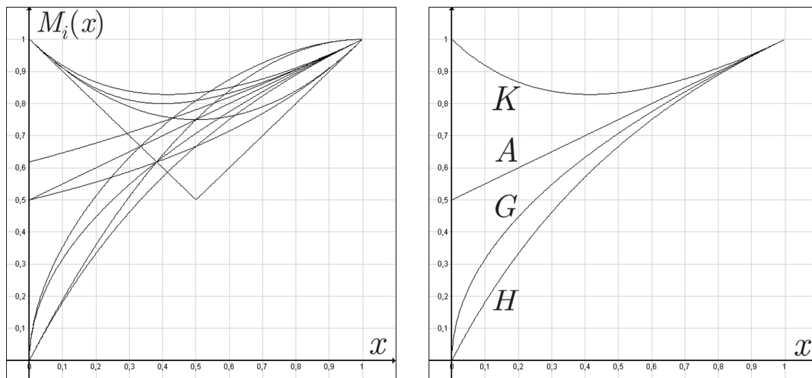
Abb. 4: pythagoreische Mittelwerte in der Reduktion auf „einstellige“ Funktionen x \mapsto M_i(x, 1) für 0 \leq x \leq 1 ; links alle, rechts auszugsweise die drei klassischen Mittelwerte und das kontraharmonische Mittel. 18
