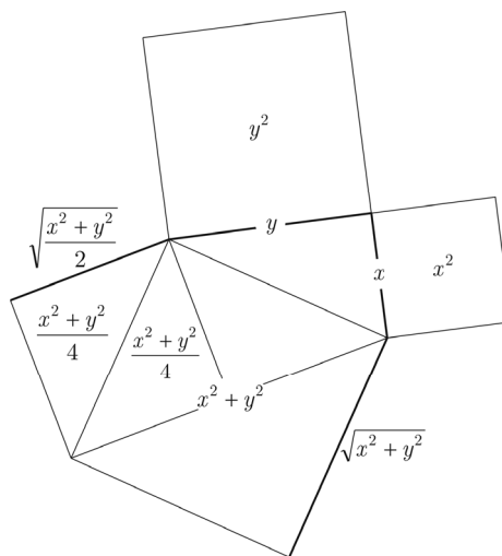
Abb. 14: Zur Konstruktion des quadratischen Mittels
