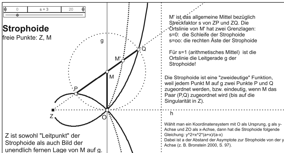
Abb. 23: Zum Entstehungsprozess des Zusammenhangs zwischen Mittelwerten und der Strophoide
