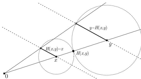
Abb. 12: harmonisches Mittel und harmonische Teilung
