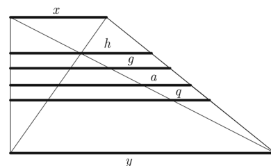
Abb. 16: Darstellung von Mittelwerten durch Mittelparallelen
