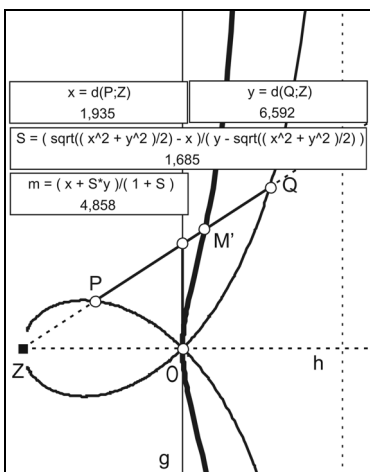
Abb. 27: strophoidale Darstellung für das quadratische Mittel
