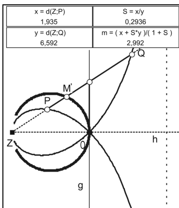
Abb. 24: strophoidale Darstellung für das harmonische Mittel
