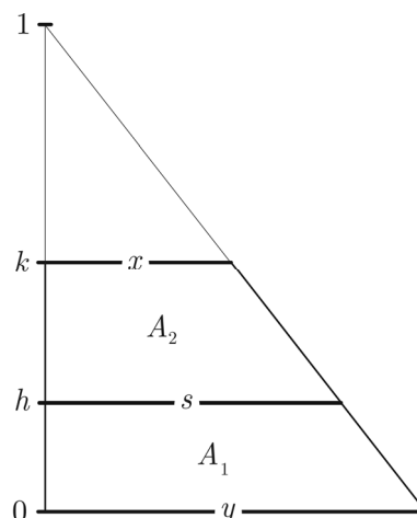
Abb. 18: Quadratmittel als Mittellinie – zum Beweis
