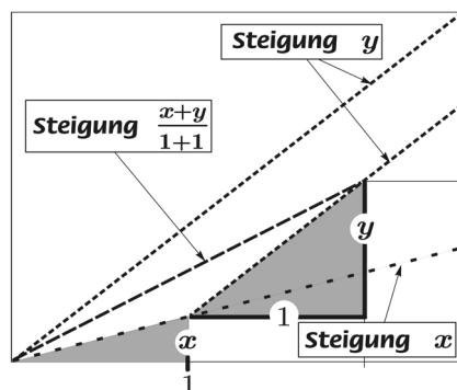
Abb. 7: Chuquetmittel von x und y ?
