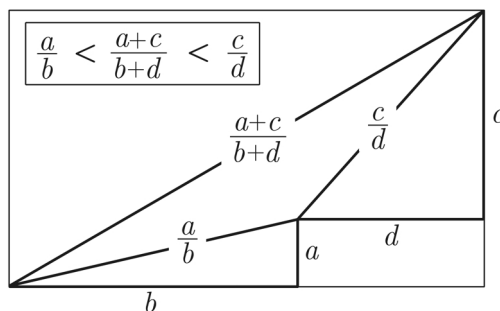
Abb. 6: Visualisierung des Chuquet-Mittels
