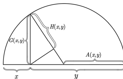
Abb. 5: Visualisierung der babylonischen Ungleichungskette nach Pappus
