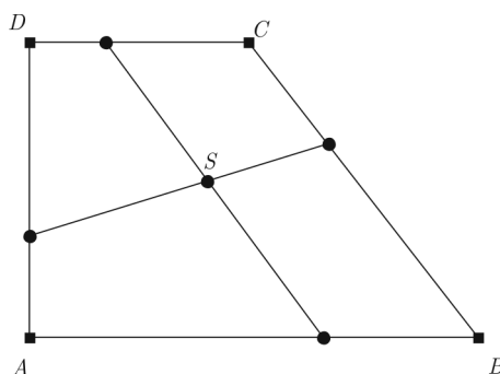
Abb. 19: Variation des Transversalenschnittkreuzes
